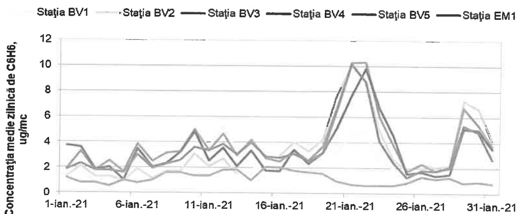
Figura 1.1.2.6.1: Evoluția mediilor zilnice de benzen în luna ianuarie
