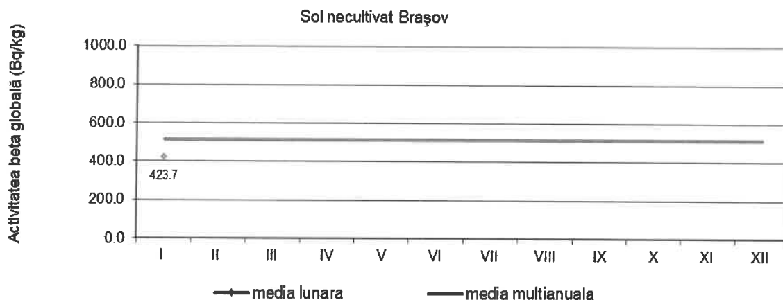
Fig. 1.3.8. Activitatea beta globală la 5 zile pentru solul necultivat
