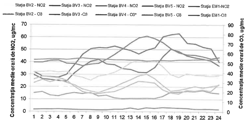
Figura 1.1.2.3.3. Ciclul zilnic al O 3 și NO 2
