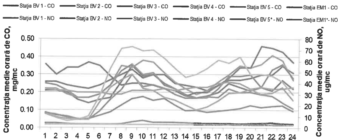
Figura 1.1.2.2.4. Ciclu zilnic al NO și CO
