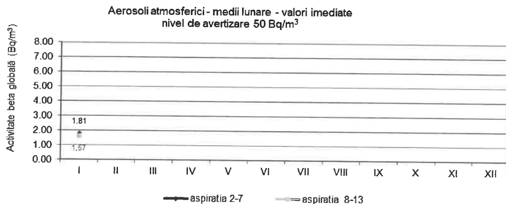
Fig. 1.3.1. Activitatea beta globală pentru aerosoli atmosferici
