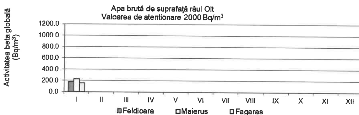
Fig. 1.3.7. Activitatea beta globală la 5 zile pentru apa de suprafață Râul Olt
